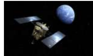
はやぶさ2
